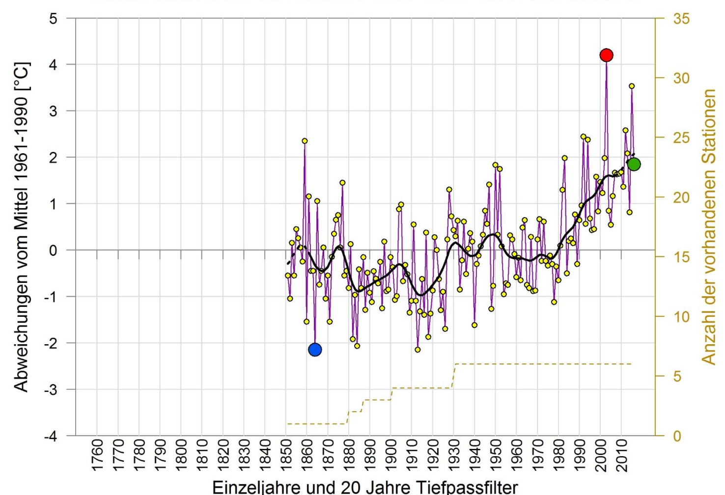
SOMMERMITTELTEMPERATUR 1851 - 2016 GIPFELREGIONEN
