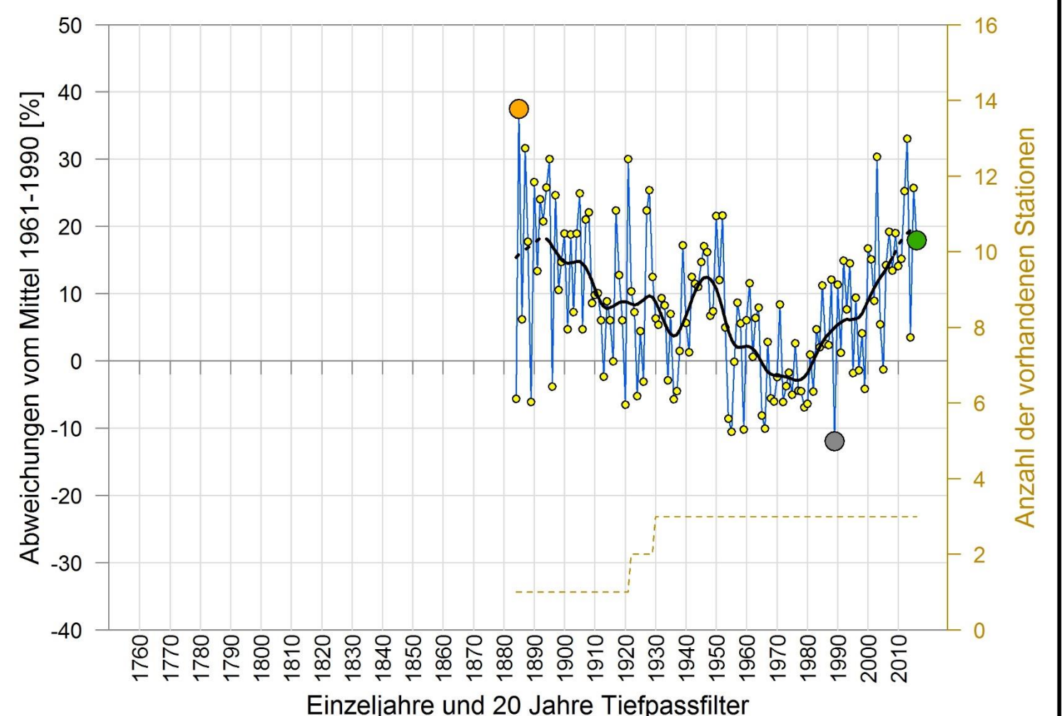
SOMMERSONNENSCHENITREIHEN 1884 - 2016 REGION SÜDOST
