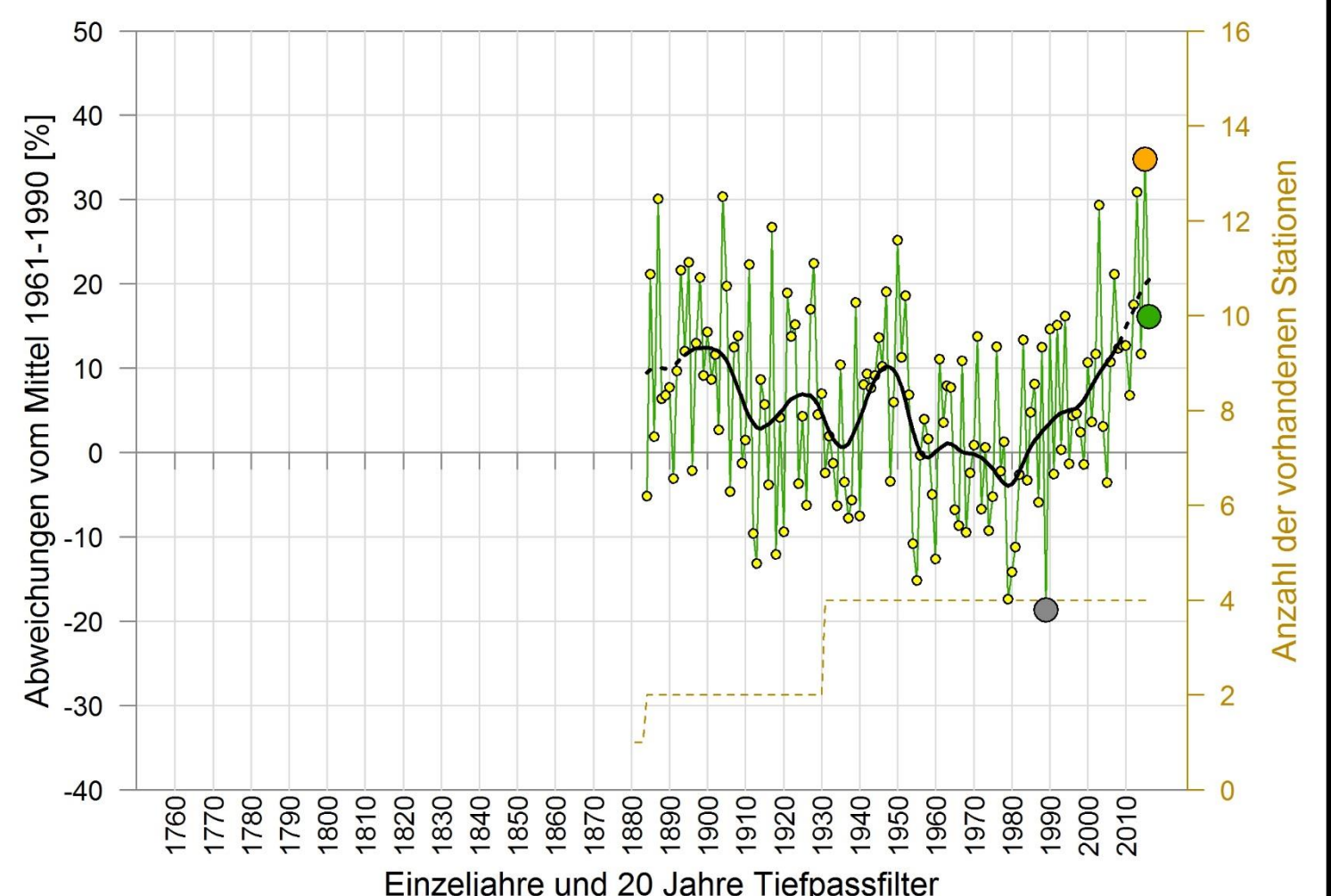
SOMMERSONNENSCHENITREIHEN 1884 - 2016 REGION NORD
