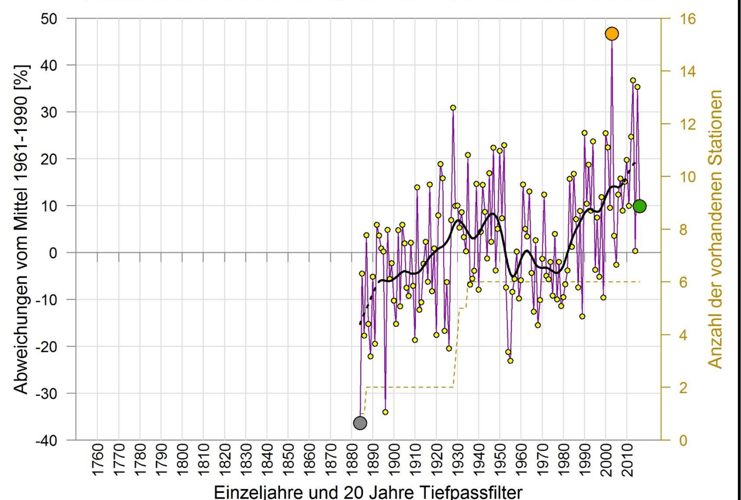
SOMMERSONNENSCHENITREIHEN 1884 - 2016 GIPFELREGIONEN
