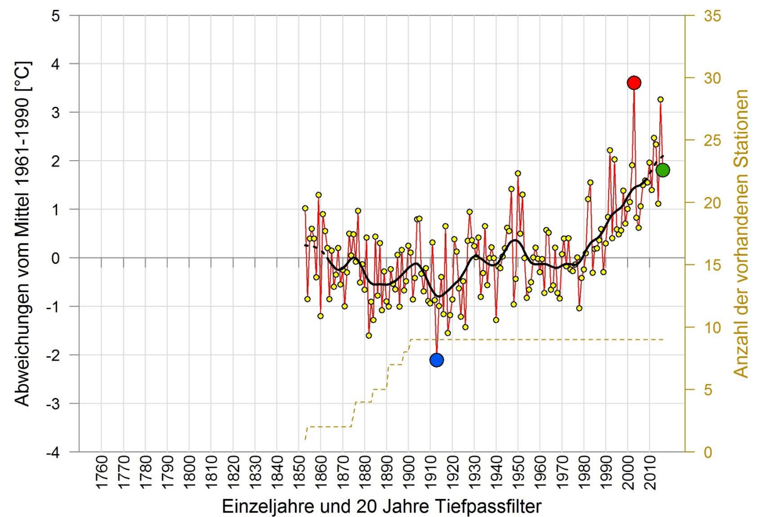
SOMMERMITTELTEMPERATUR 1853 - 2016 REGION INNERALPIN
