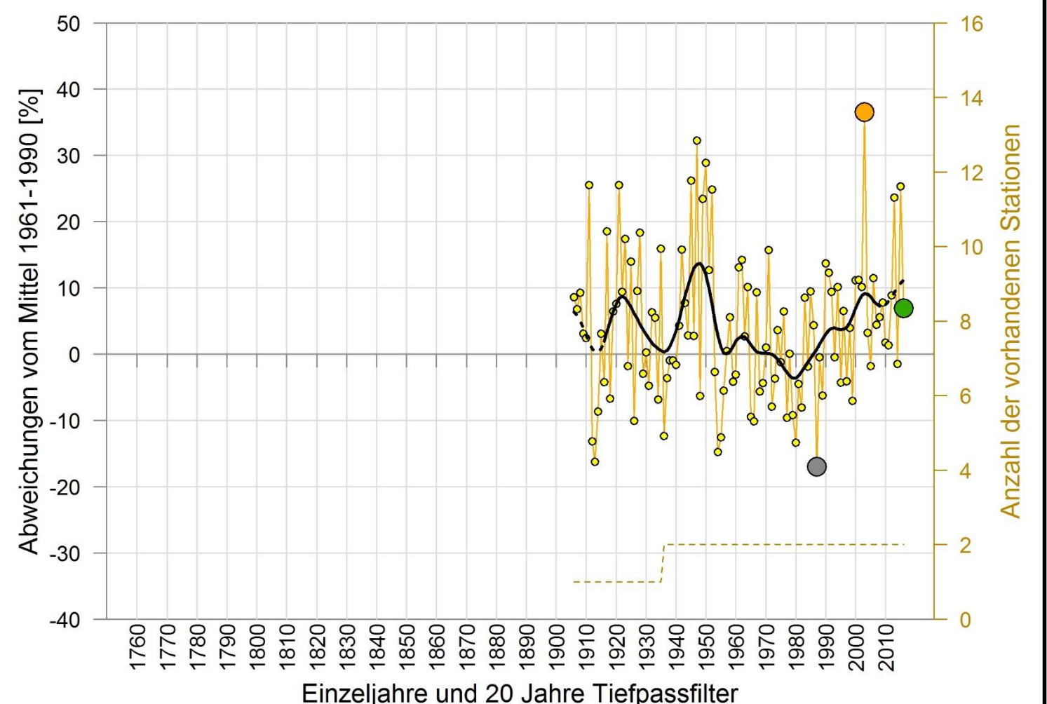
SOMMERSONNENSCHENITREIHEN 1906 - 2016 REGION WEST
