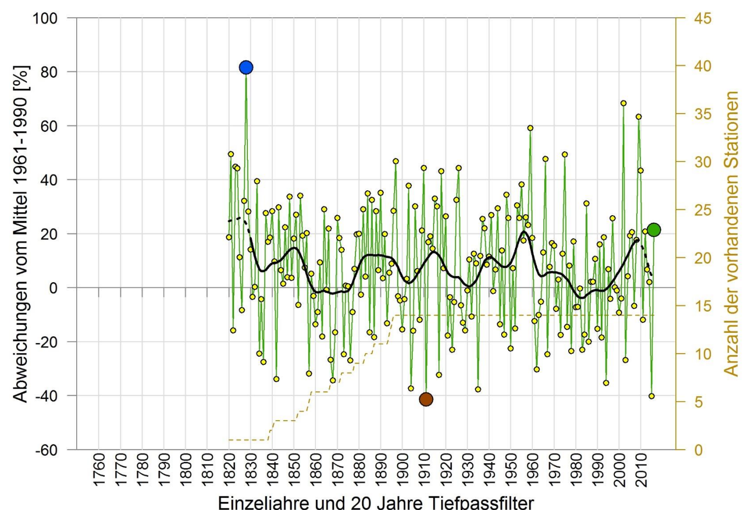
SOMMERNIEDERSCHLAG 1820 - 2016 REGION NORD
