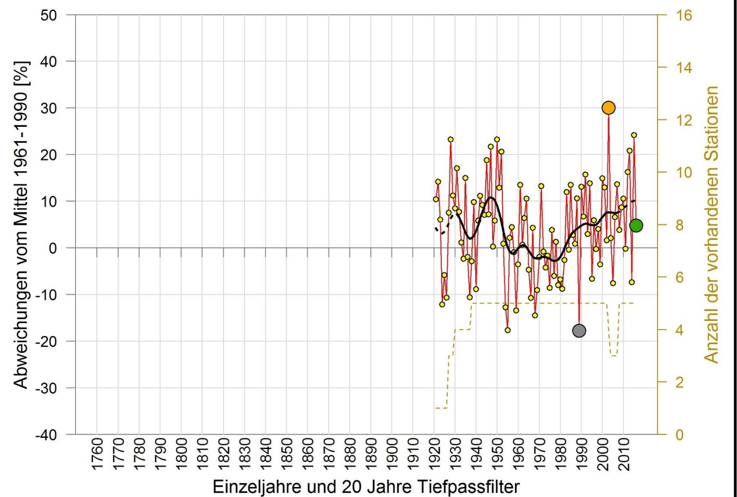
SOMMERSONNENSCHENITREIHEN 1921 - 2016 REGION INNERALPIN
