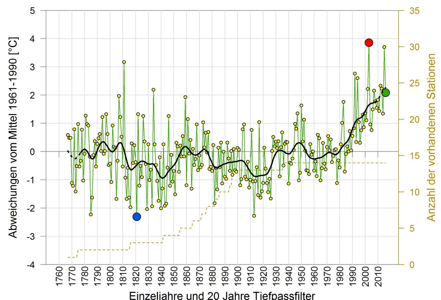
SOMMERMITTELTEMPERATUR 1767 - 2016 REGION NORD
