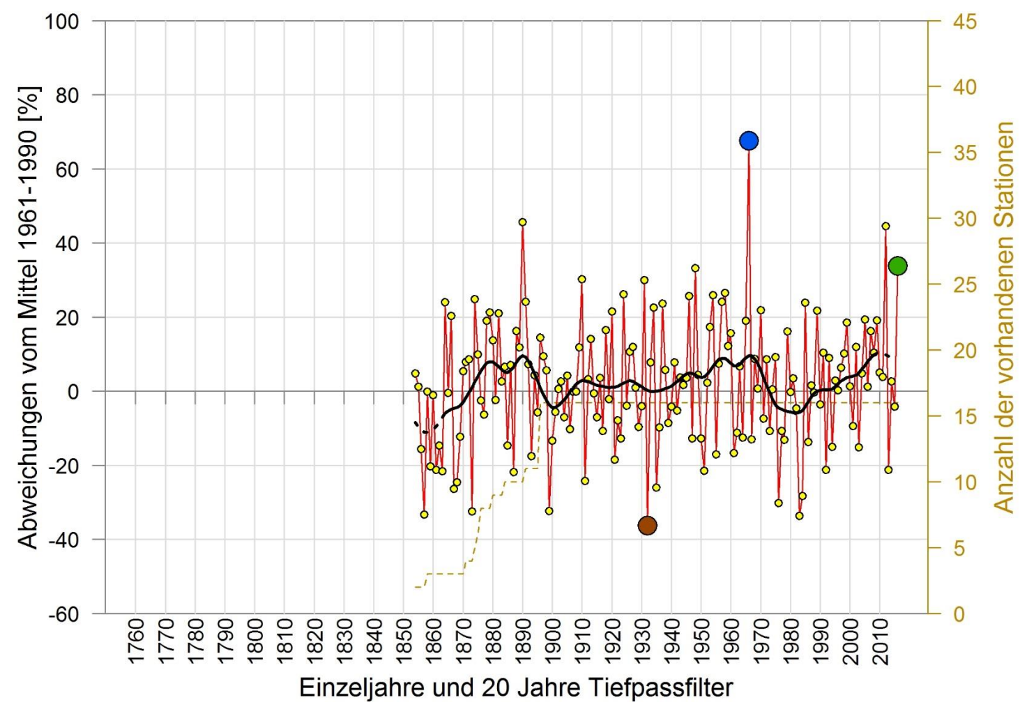
SOMMERNIEDERSCHLAG 1854 - 2016 REGION INNERALPIN
