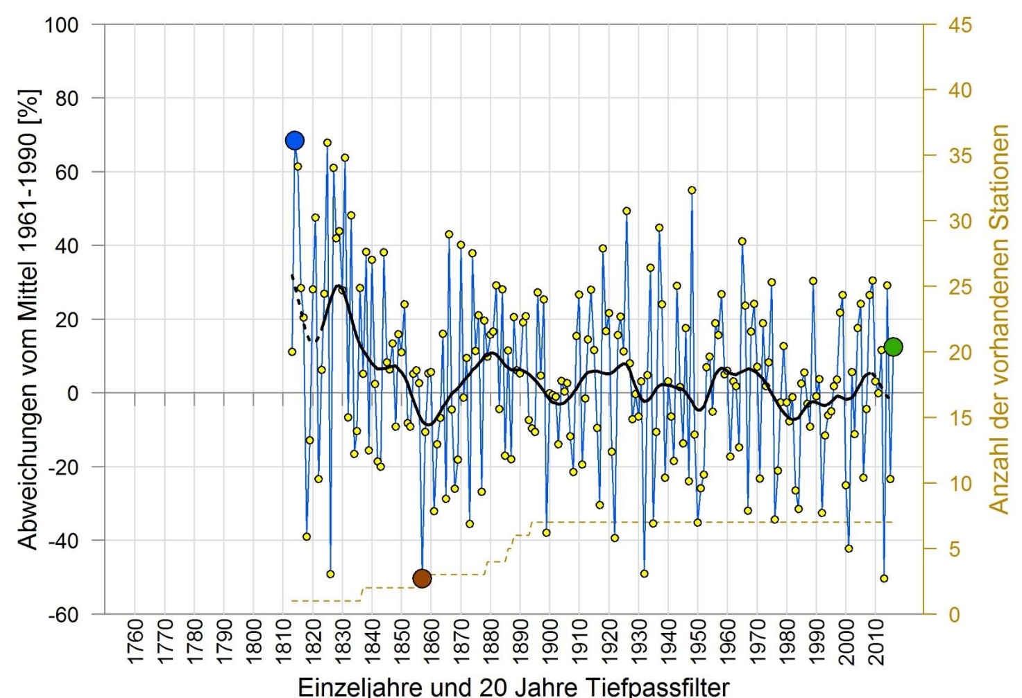
SOMMERNIEDERSCHLAG 1813 - 2016 REGION SÜDOST
