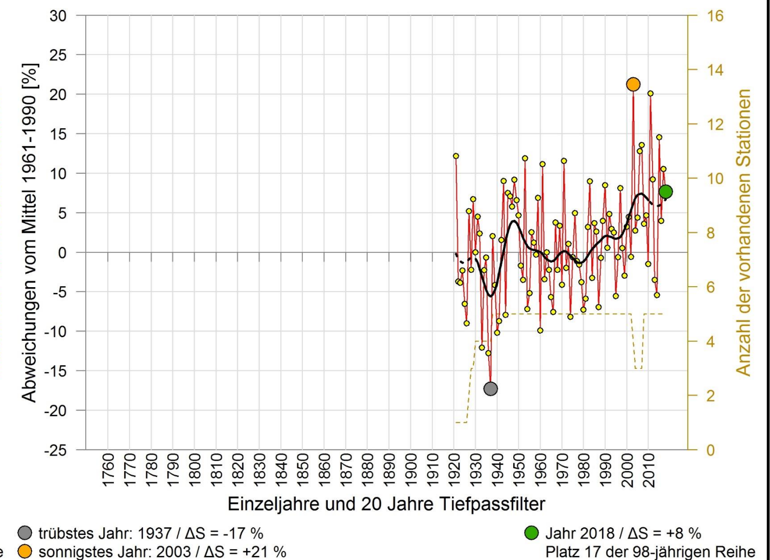
JAHRESSONNENSCHINDAUER 1921 - 2018 REGION INNERALPIN
