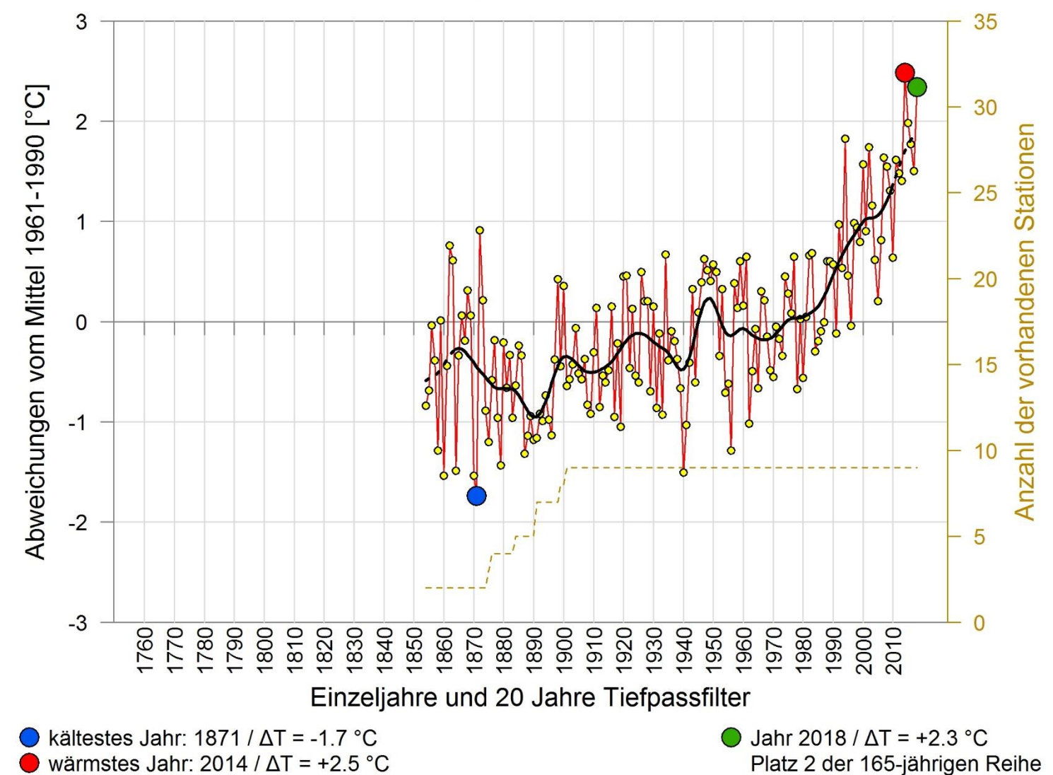
JAHRESMITTELTEMPERATUR 1854 - 2018 REGION INNERALPIN
