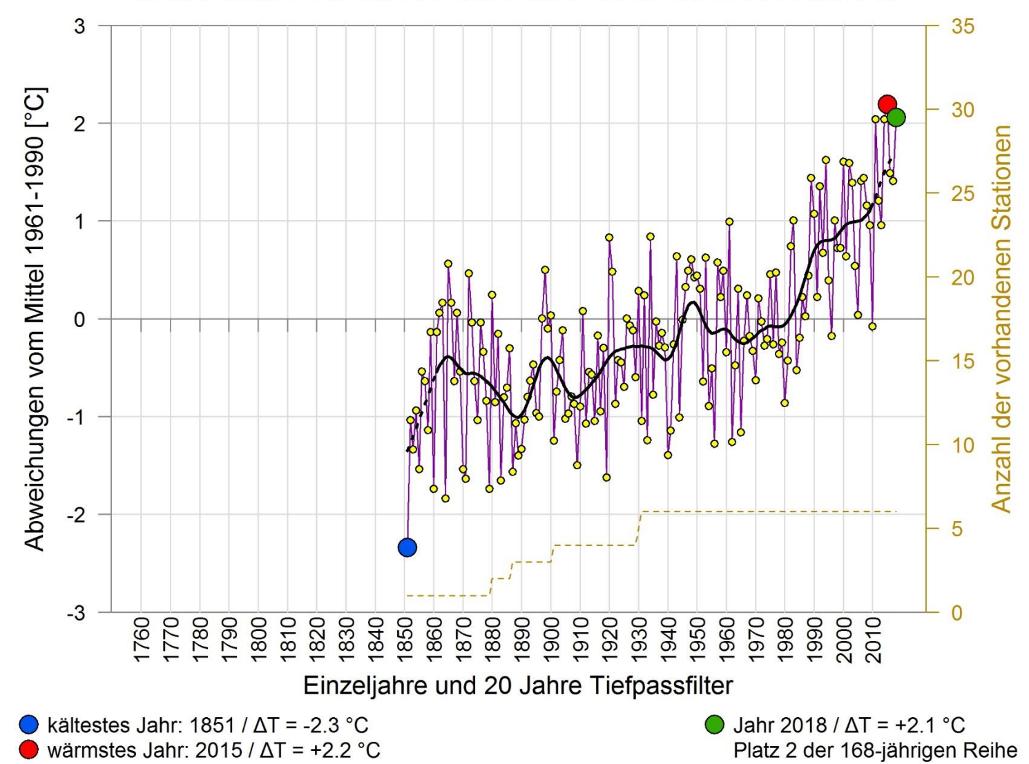
JAHRESMITTELTEMPERATUR 1851 - 2018 GIPFELREGIONEN
