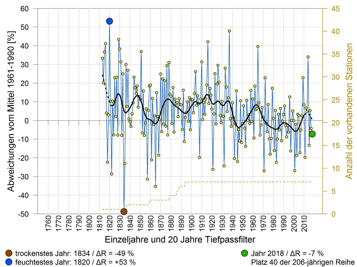
JAHRESNIEDERSCHLAG 1813 - 2018 REGION SÜDOST
