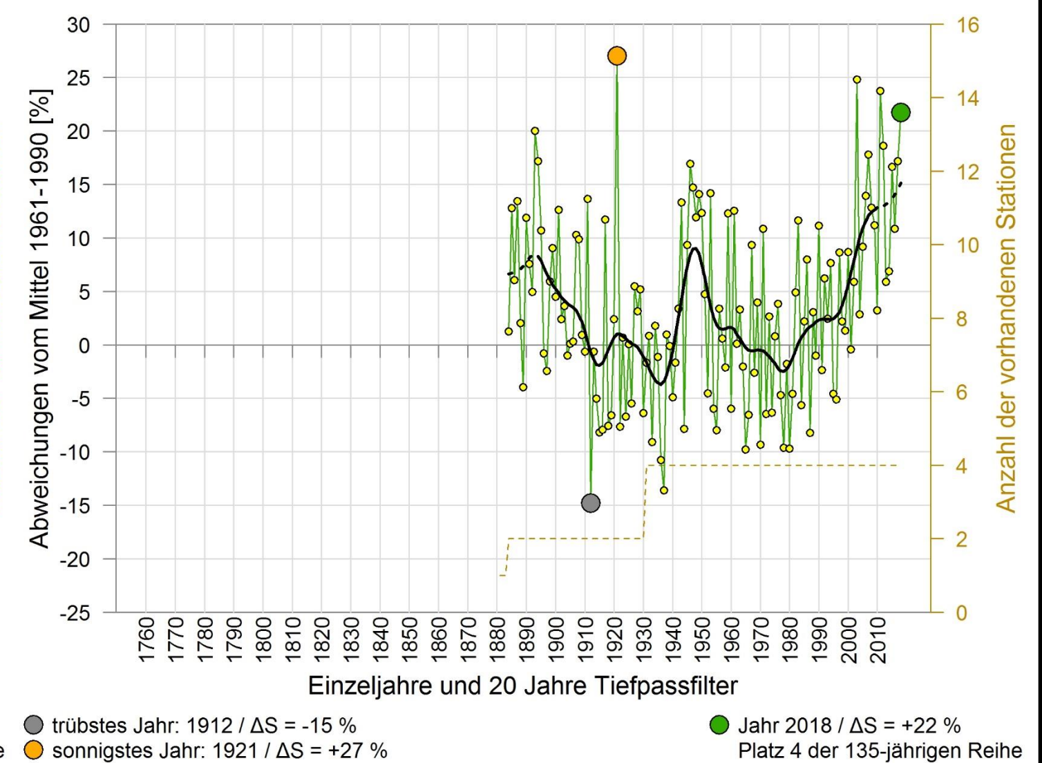
JAHRESSONNENSCHINDAUER 1884 - 2018 REGION NORD
