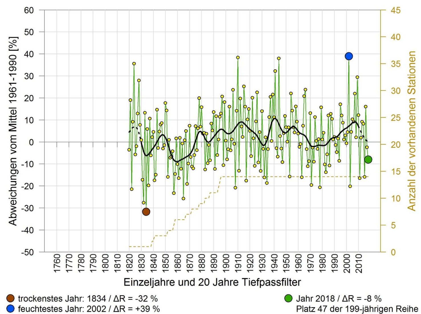
JAHRESNIEDERSCHLAG 1820 - 2018 REGION NORD
