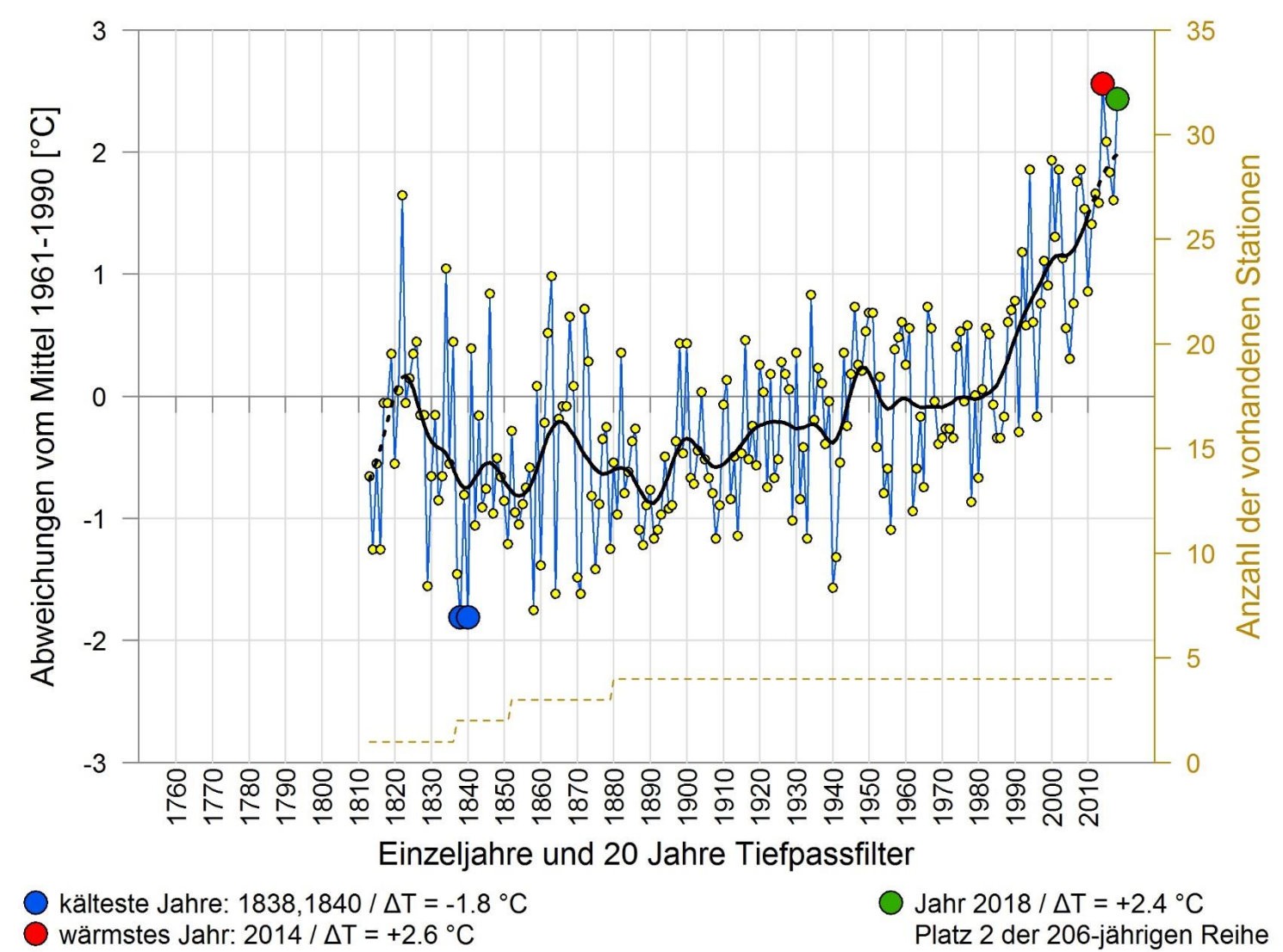
JAHRESMITTELTEMPERATUR 1813 - 2018 REGION SÜDOST
