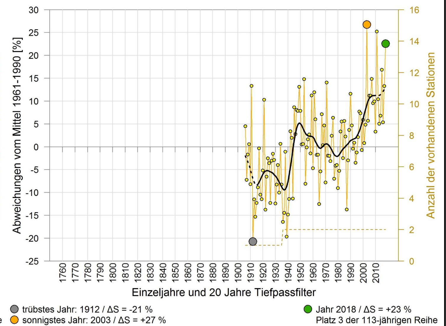
JAHRESSONNENSCHINDAUER 1906 - 2018 REGION WEST
