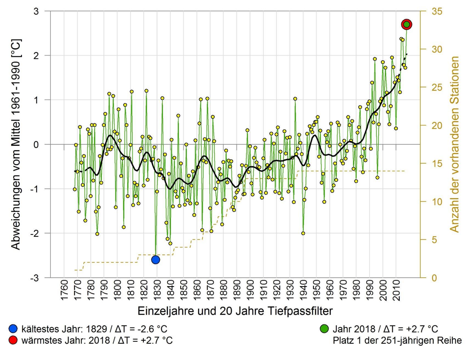
JAHRESMITTELTEMPERATUR 1768 - 2018 REGION NORD
