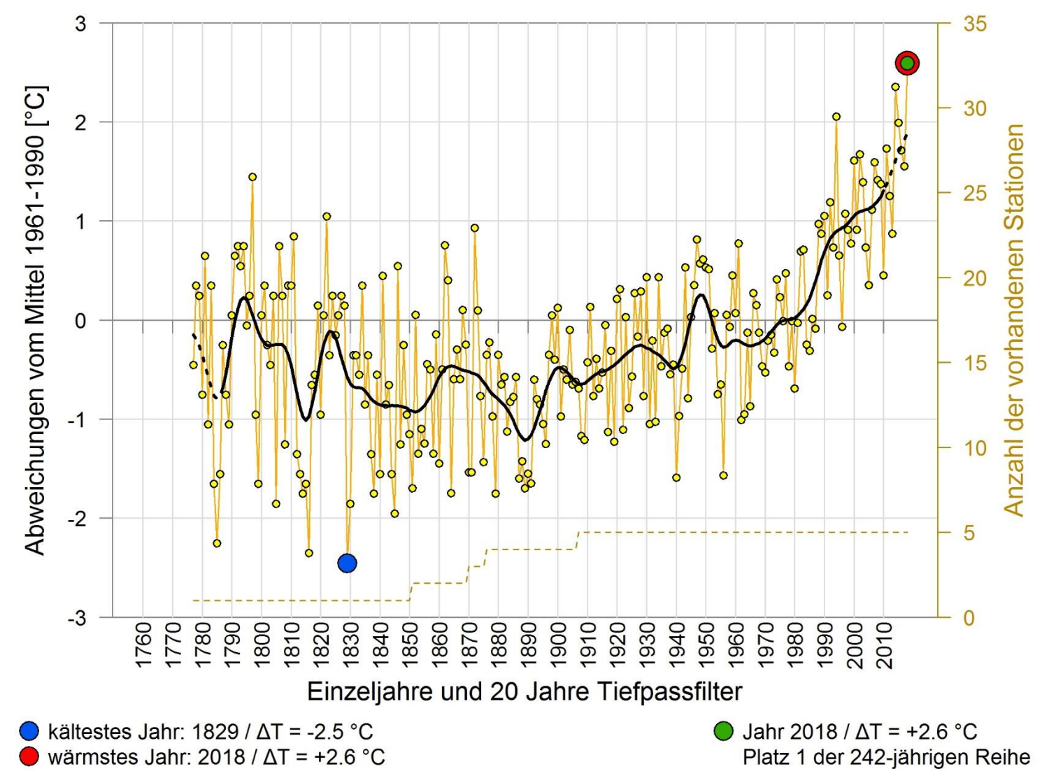
JAHRESMITTELTEMPERATUR 1777 - 2018 REGION WEST
