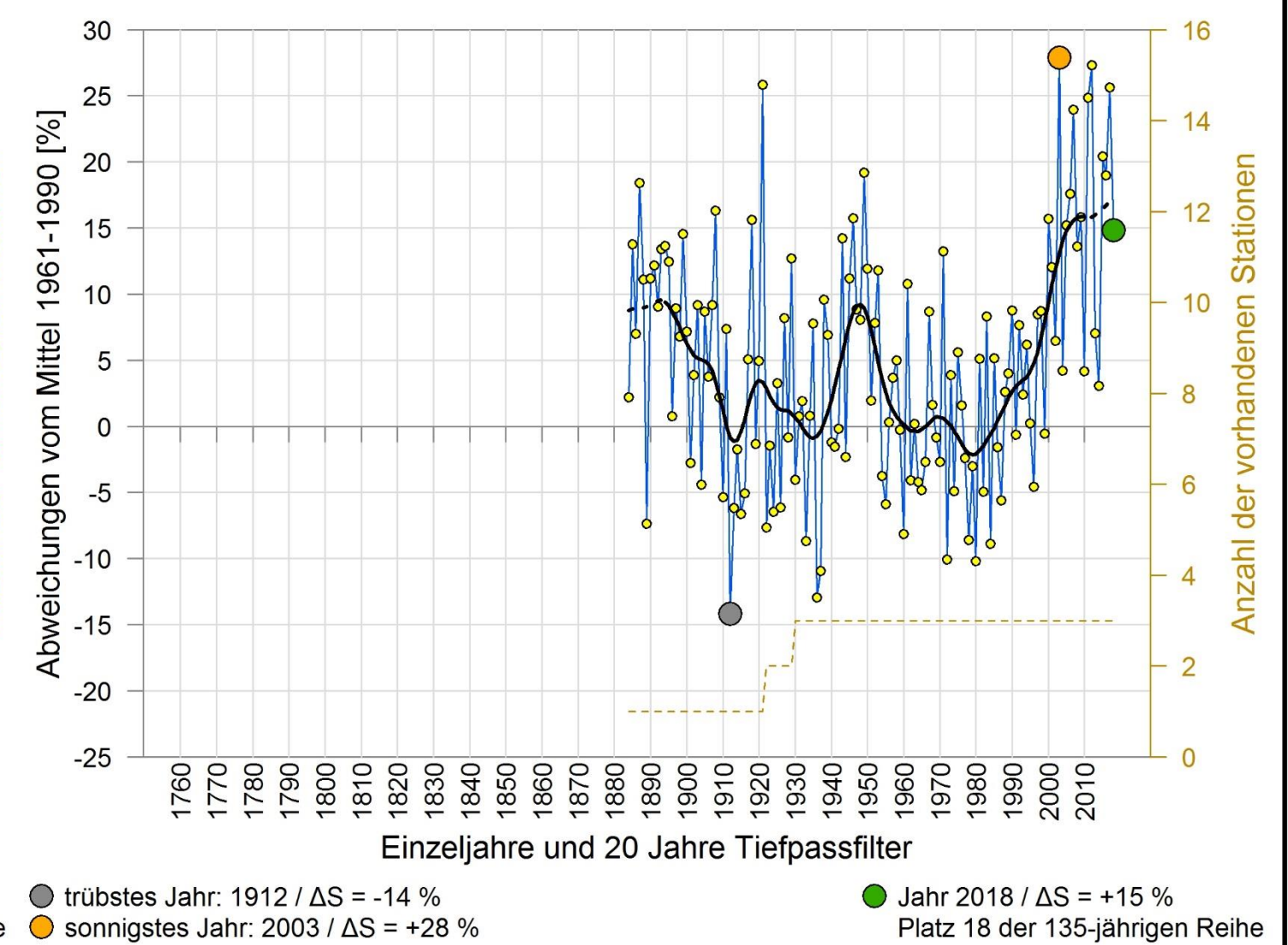
JAHRESSONNENSCHINDAUER 1884 - 2018 REGION SÜDOST
