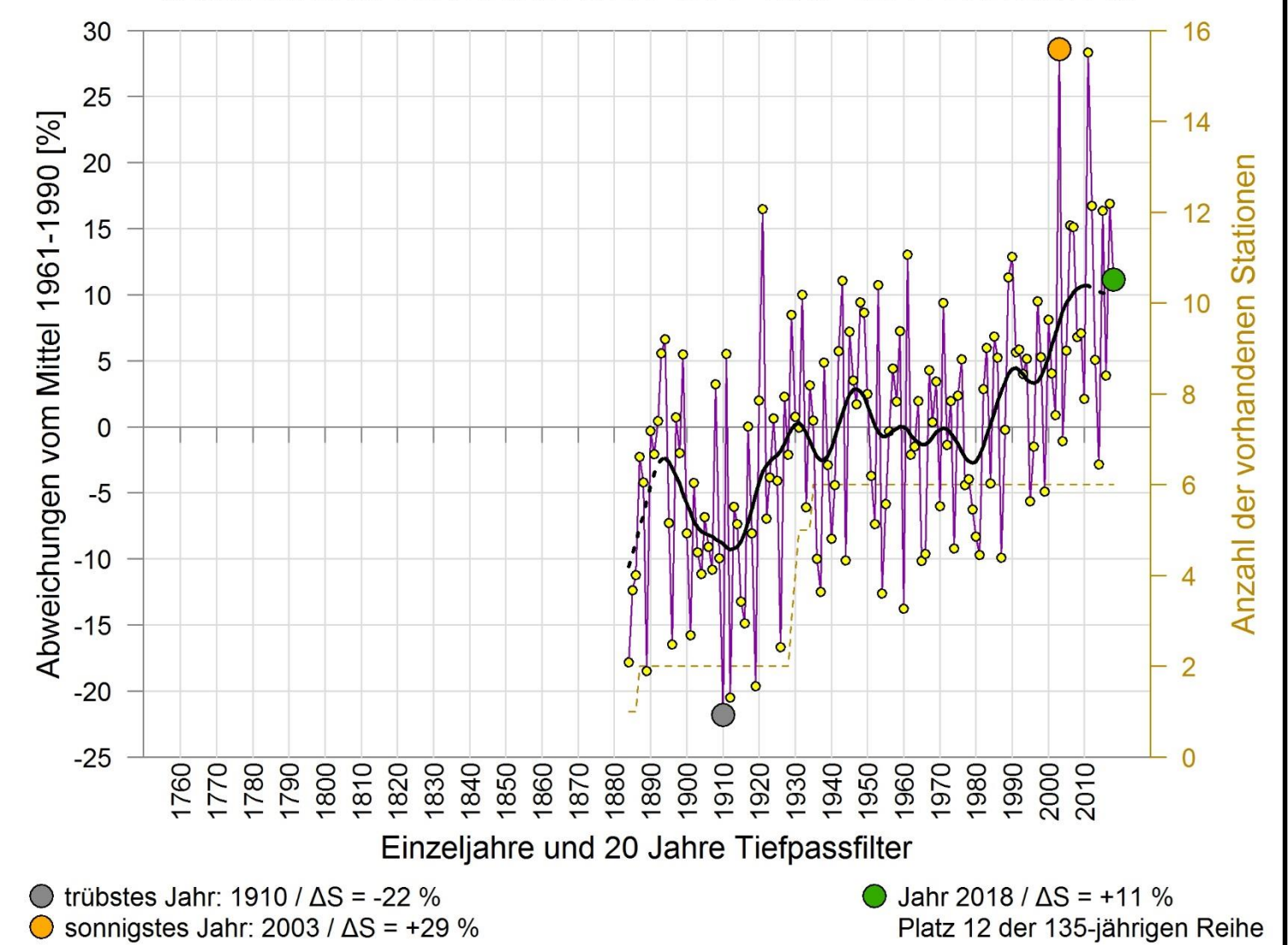
JAHRESSONNENSCHINDAUER 1884 - 2018 GIPFELREGIONEN
