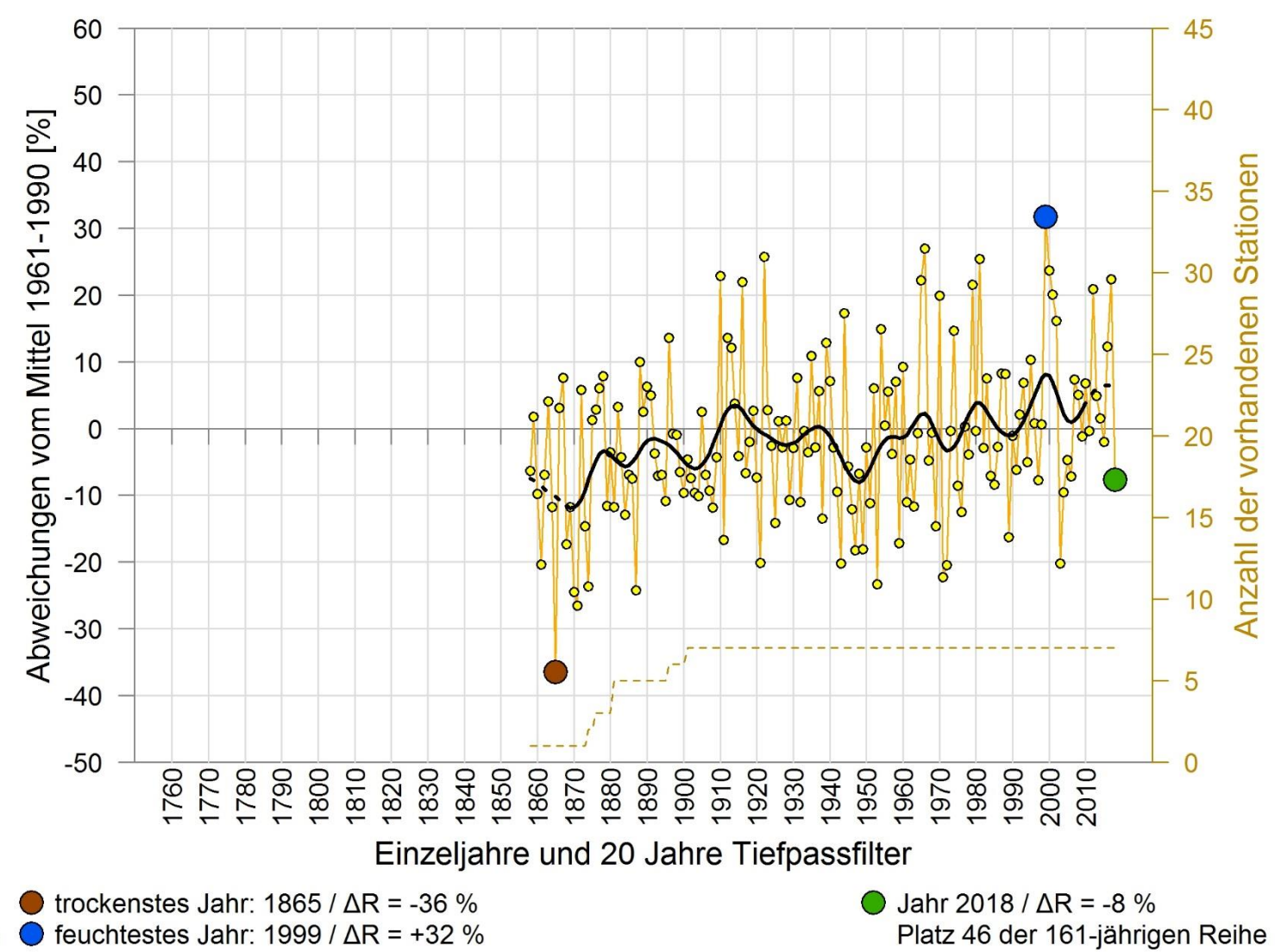
JAHRESNIEDERSCHLAG 1858 - 2018 REGION WEST
