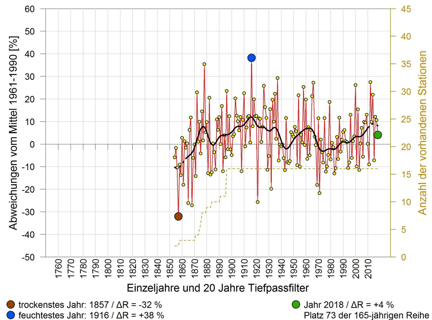
JAHRESNIEDERSCHLAG 1854 - 2018 REGION INNERALPIN
