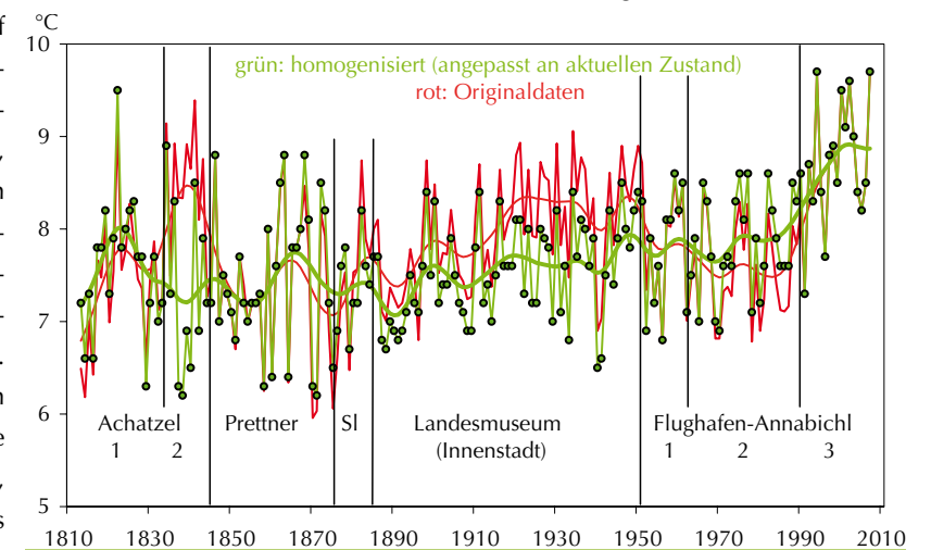
Abb. 2: Die Temperaturreihe von Klagenfurt 1813-2007, die aus verschiedenen Einzelreihen zusammengesetzt wurde. Gezeigt sind die Jahresmittel und der 30-jährig geglättete Verlauf (Gauß'scher Tiefpassfilter) der Originaldaten (rot) und die homogenisierte Reihe, die an den aktuellen Zustand (seit 1991) einer automatischen Messstation auf dem Flughafen angepasst ist. Quelle: Version 2008 der HISTALP-Datenbank der ZAMG; AUER et al., 2007, BÖHM, 2009a
