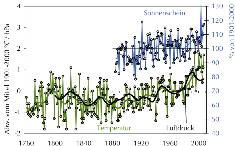
Abb. 5: Jahresmittelreihen von drei eng gekoppelten Klimaelementen im Großraum Alpen. Grün: Lufttemperatur (Mittel aller Tieflandstationen, Einzeljahre und 30-jährig geglättet), schwarz: Luftdruck (Mittel aller Tieflandstationen, nur die geglättete Kurve gezeigt), blau: hochalpines Mittel der Sonnenscheindauer (Einzeljahre und 30-jährig geglättet)
