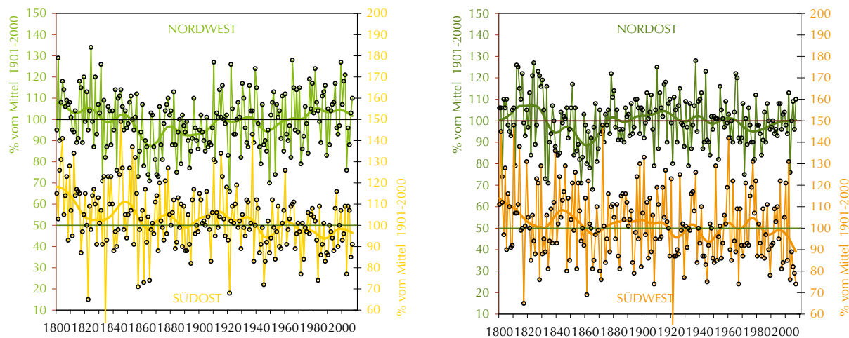
Abb. 6: Regionale Jahressummenreihen 1800–2007 des Niederschlages im Großraum Alpen. Links: CRS-Nordwest (grün) und CRS-Südost (gelb), rechts: CRS-Nordost (grün) und CRS-Südwest (orange). Einzeljahre und 30-jährig geglätteter Verlauf (Gauß'scher Tiefpassfilter), Relativwerte (in Prozent des Mittels des 20. Jahrhunderts)
