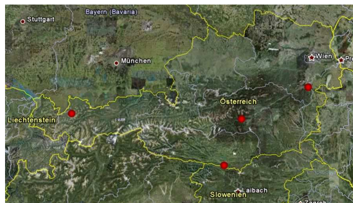
Lage der verspürten Erdbeben in Österreich im August 2011 (Bildmaterial: Google Earth Pro)
